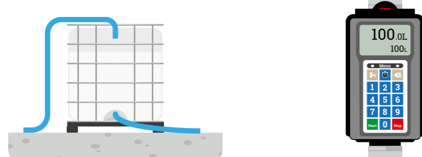
Citerne intermédiaire : vol max = vol cuve
