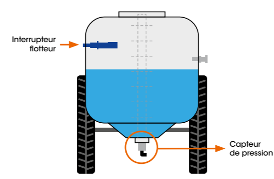
Arrêt automatique : jauge / capteur électronique, ...
